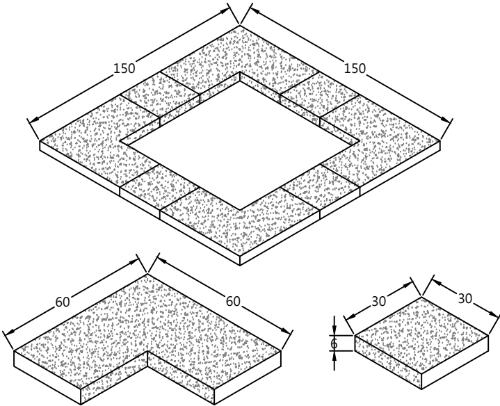
預鑄洗石子(噴砂)樹穴(W=30cm)
